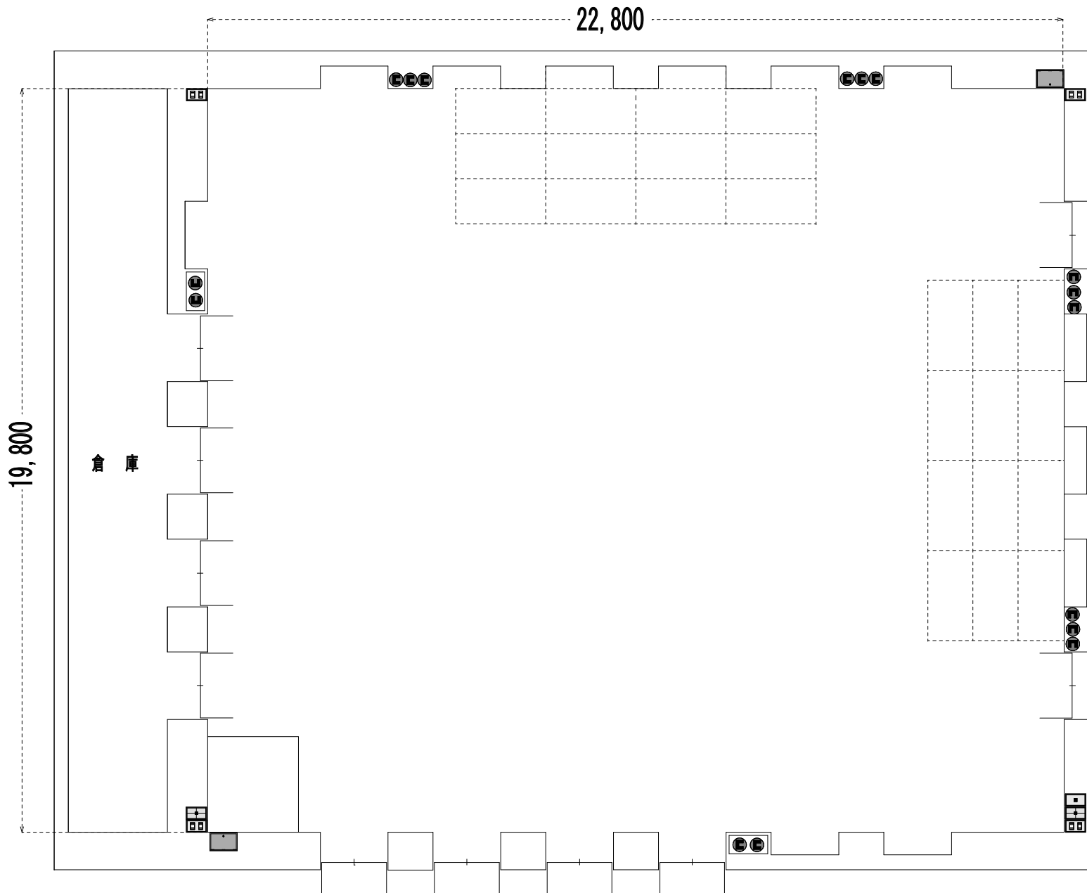
中ホール平面図【設備表示】
